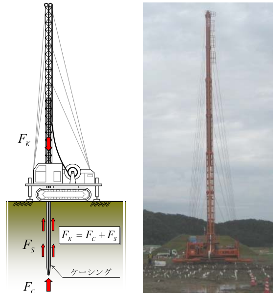
図1 力の釣合い
