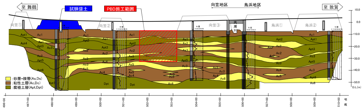
図 13 向笠地区の地質想定縦断面図
