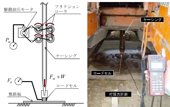
図3 打設力検定試験
