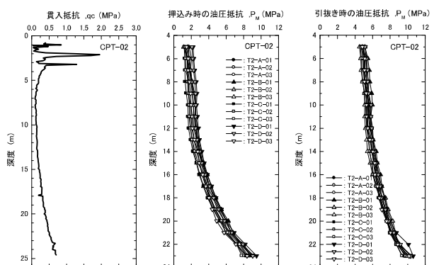
図6 コーン貫入試験結果 (CPT-02)
