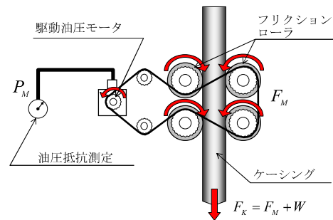
図2 ケーシング貫入機構の模式図
