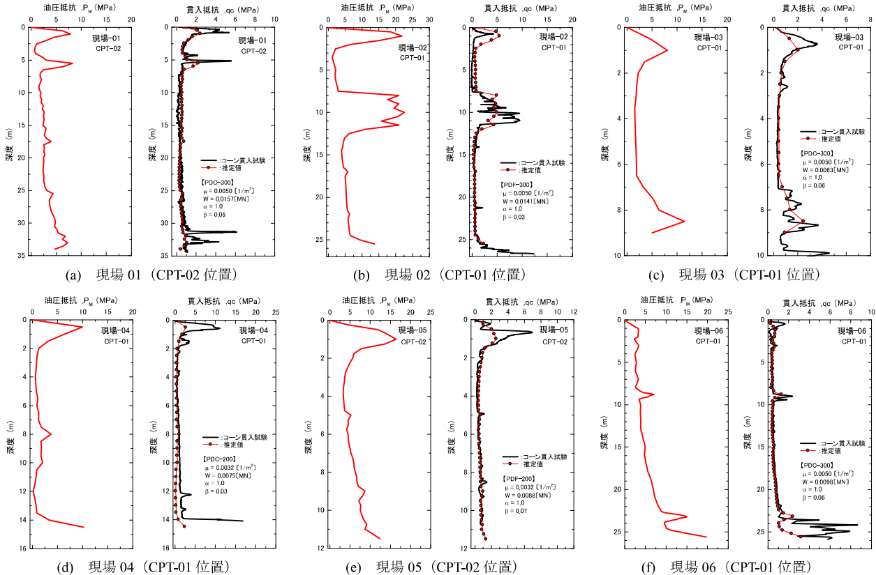
図10 ケーシングの押し込み・引き抜き試験による油圧抵抗深度分布
