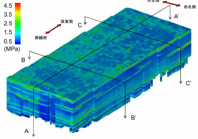
図 16 推定した貫入抵抗の分布 (3次元)
